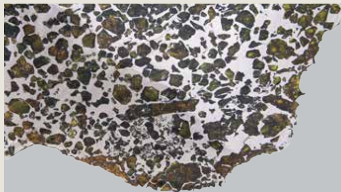
MÉTÉORITES MIXTES (1%)
