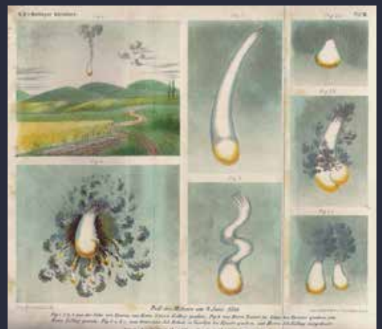
Représentation (gravure) de la chute de la météorite de Knyahinya, en 1866 – CCO
