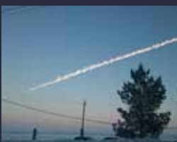
Chute de la météorite de Tcheliabinsk, en 2013 © Константин Кудинов/CC BY-SA 3.0
