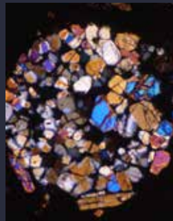
Chondre observé au microscope © M.N.H.N.
